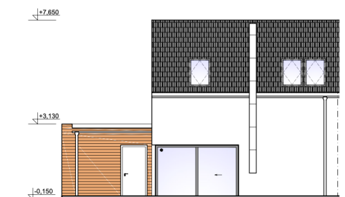
POHLED ZADNÍ:
