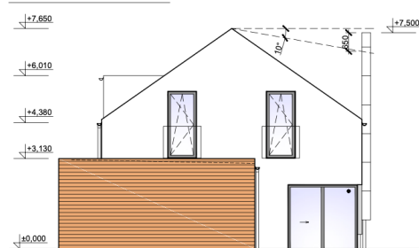
POHLED BOČNÍ:
